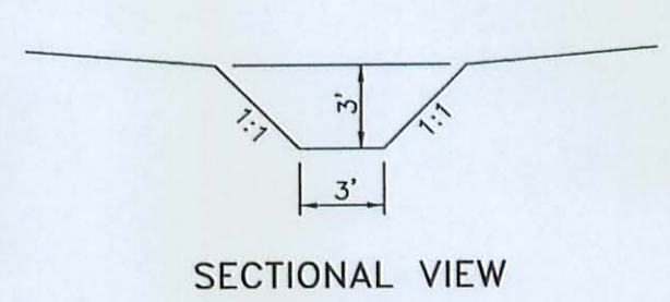
SUMP DETAIL N.T.S.
